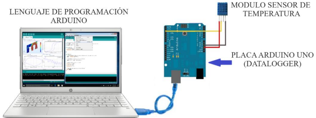
Figura 24. Conexión Arduino-PC
