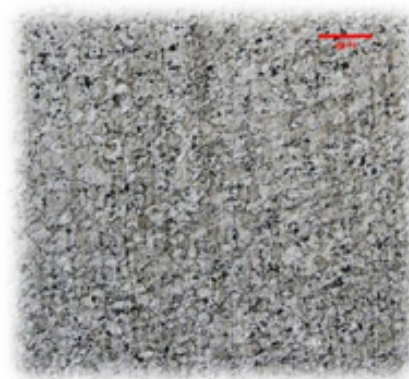
Figura 18. Fase y estructura del material base. Aumento de 100 X. Ataque con Keller.
